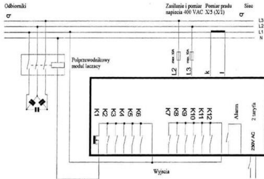
Rys.2: Schemat podłączenia dla kombinacji stycznikowych i półprzewodnikowych stopni:
