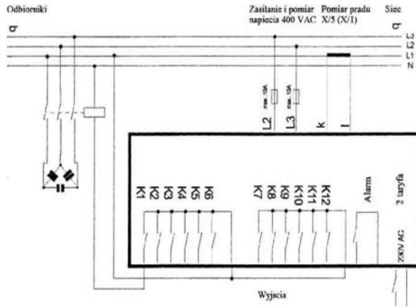
Rys.1: Schemat podłączenia ze stopniami stycznikowymi:
