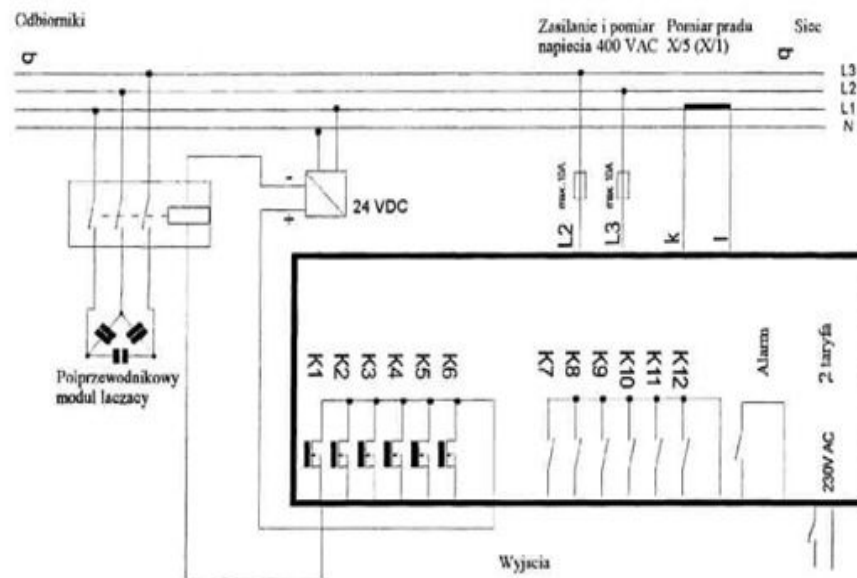
Rys.3: Schemat podłączenia regulatora z sześcioma wyjściami półprzewodnikowymi:
